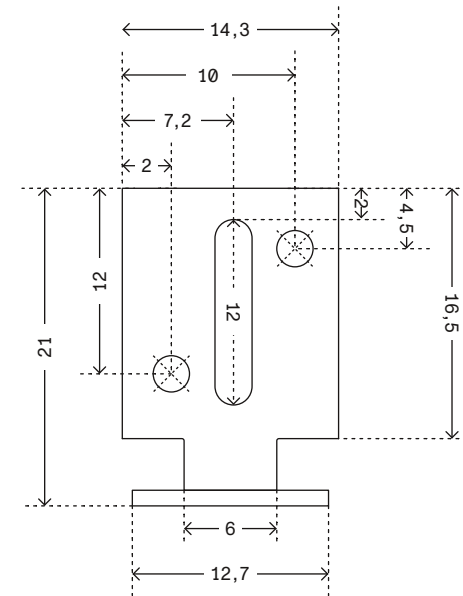
Upphängningskrok kort
