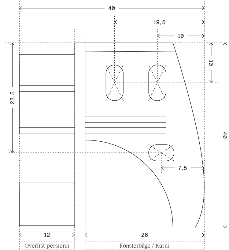
Designbeslag
