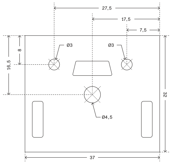
Snäppbeslag tak
