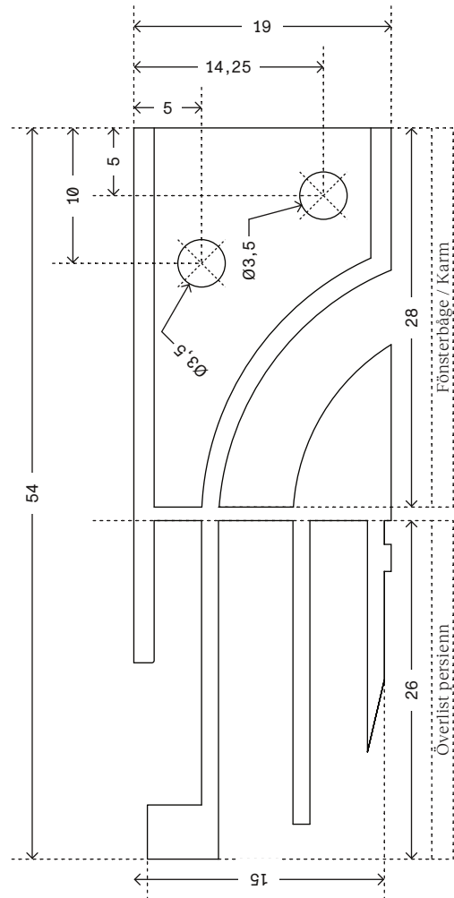
Basicbeslag
