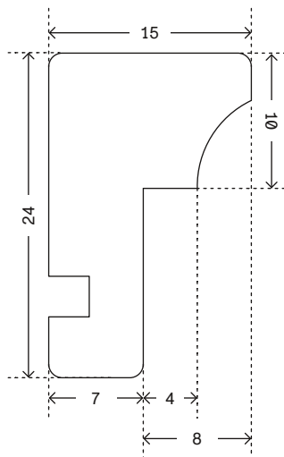
Magnethållare allmoge
