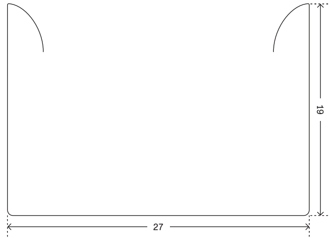
Överlist 25 mm
