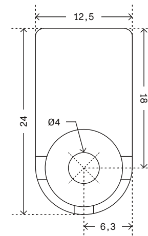
Magnethållare framifrån
