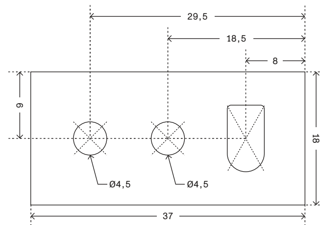
Snäppbeslag vägg
