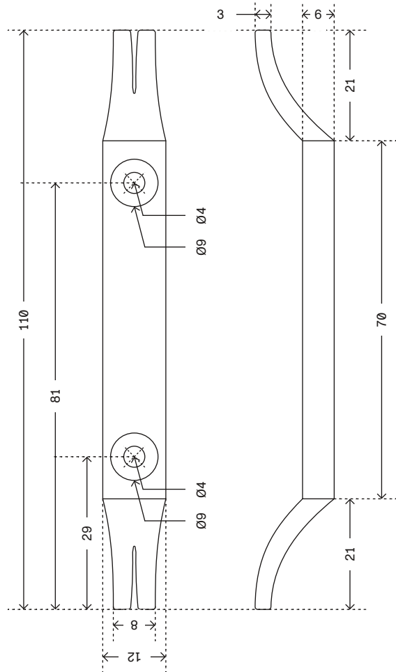
Linsamlare framifrån/sidovy
