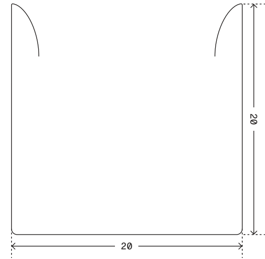
Överlist 16 mm
