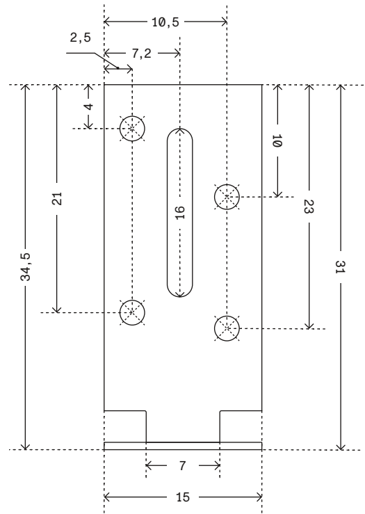
Upphängningskrok standard
