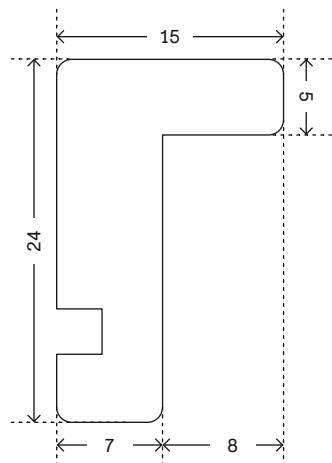
Magnethållare rak
